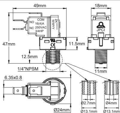
Rosca 1/4 NPSM
